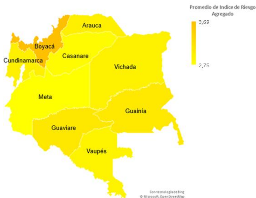
Gráfico 12. Promedio de IRA por Departamento – Orinoquía
