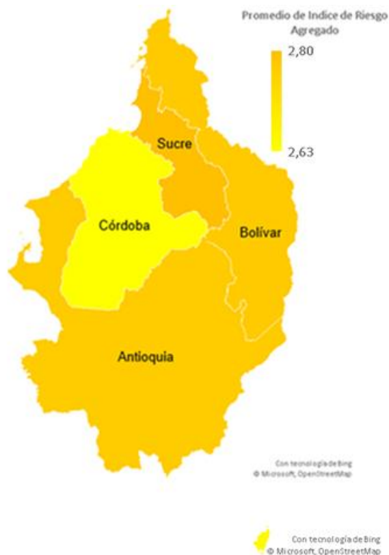
Gráfico 7. Promedio de IRA por Departamento - Costa Caribe 2
