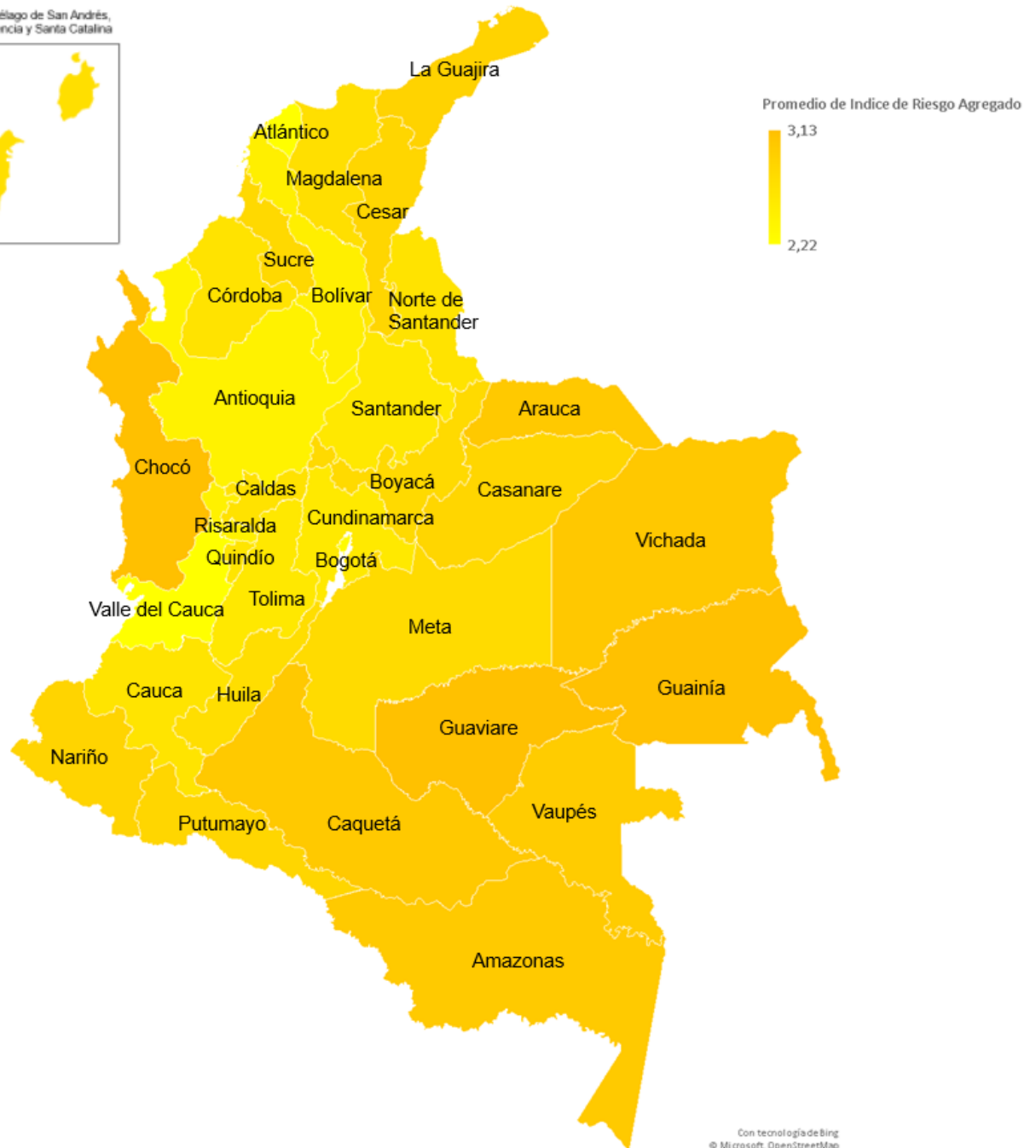
Gráfico 2. Mapa del promedio del IRA por Departamento
